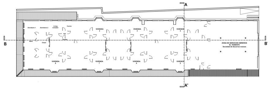
Figura 4. Secciones y planta tipo (nivel 3-4), respectivamente. Base planimétrica ente 1941 y 1950, Fundación Sewell (fuente: Elaboración propia, 2019).
