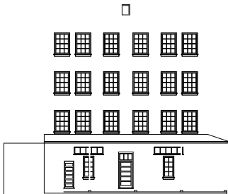
ELEVACION OESTE
